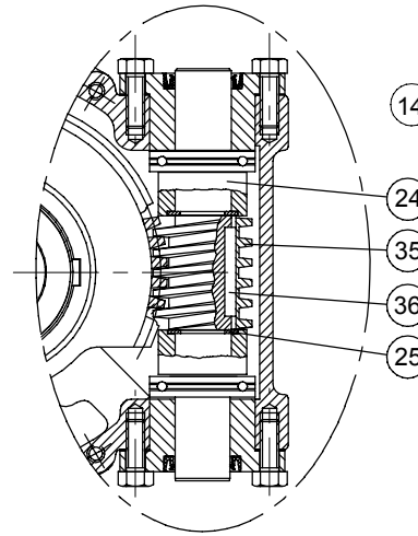
DETALLE Z DETAIL Z PARA RK-125 FOR RK-125
